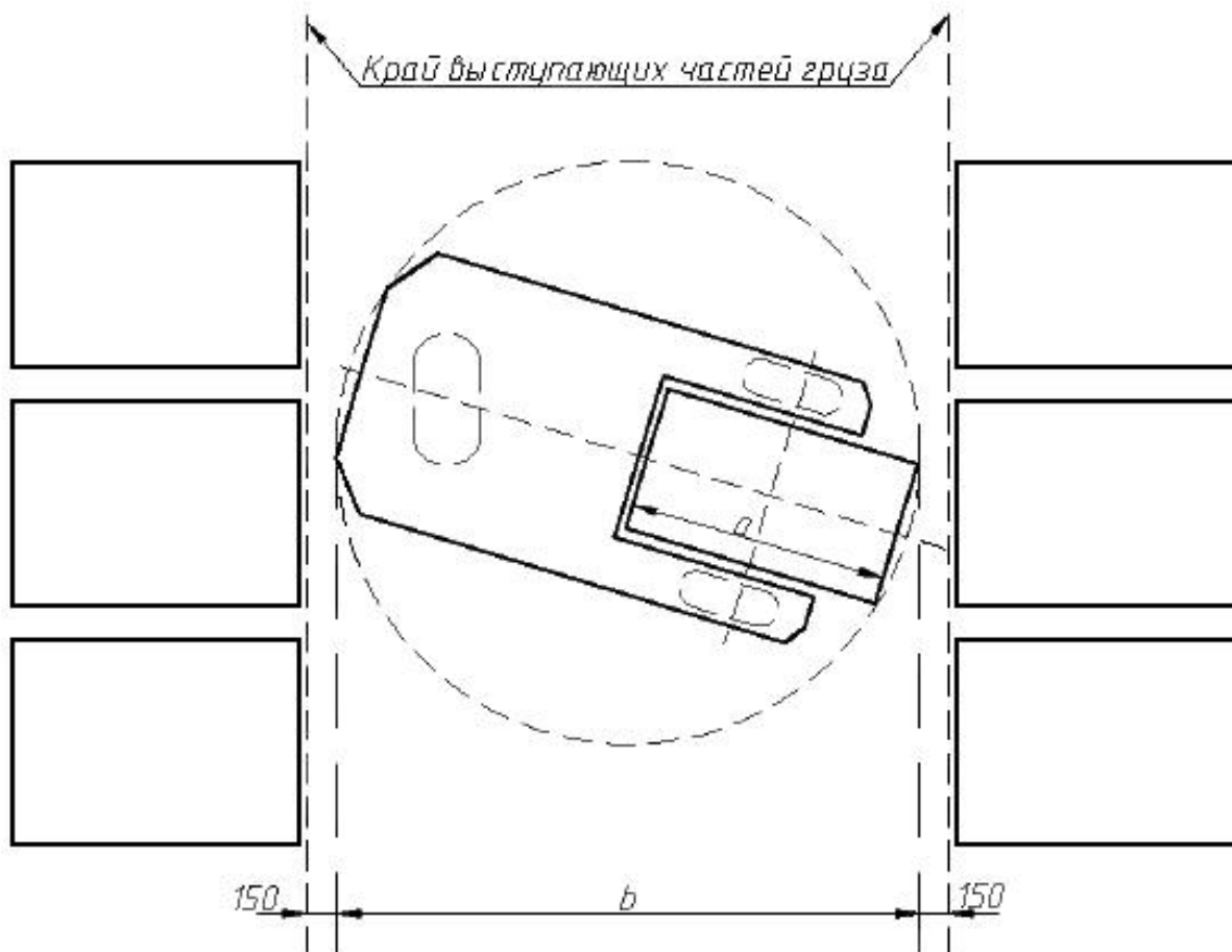
Рисунок 4 - Параметры зазора между ШТ и грузами
