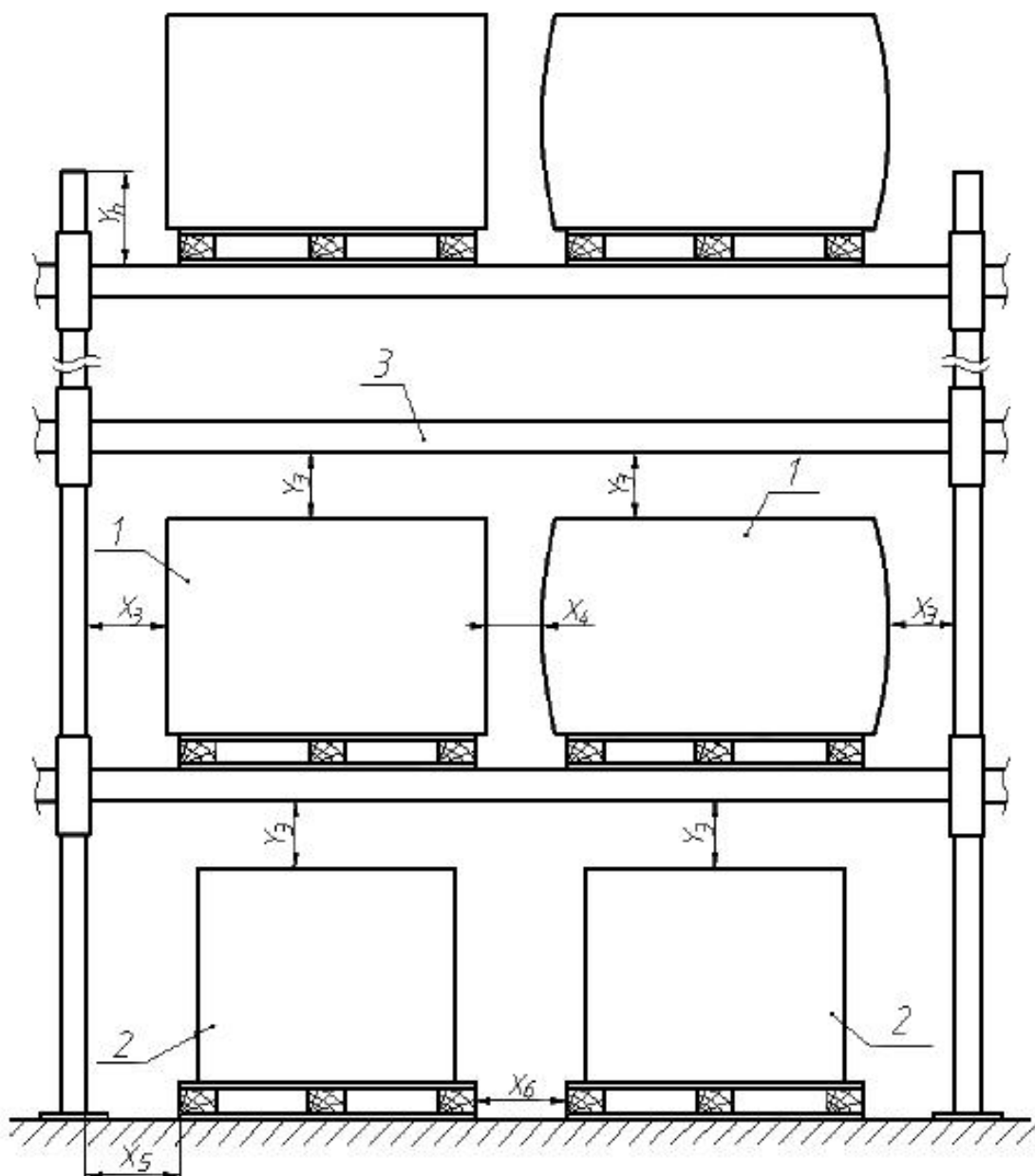
Рисунок 5 - Схема размещения груза в секции
