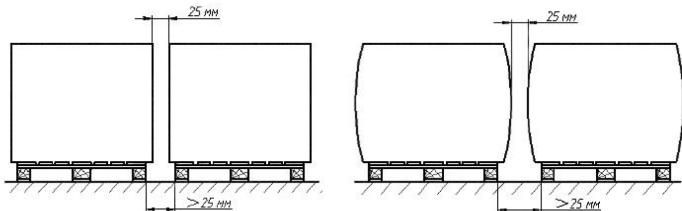
Рисунок 9 - Размещение груза в глубину канала
