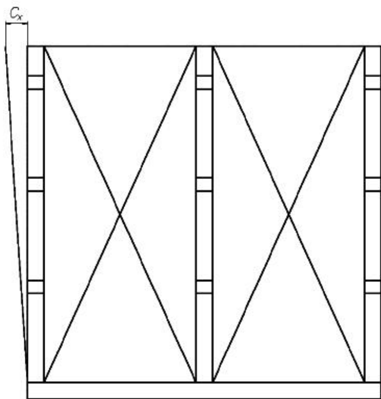
Рисунок 13 - Прогиб элементов консольных стеллажей
