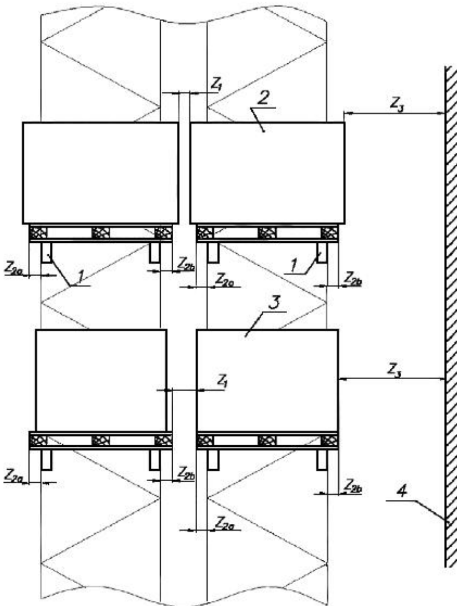
Рисунок 6 - Схема установки груза на балках
