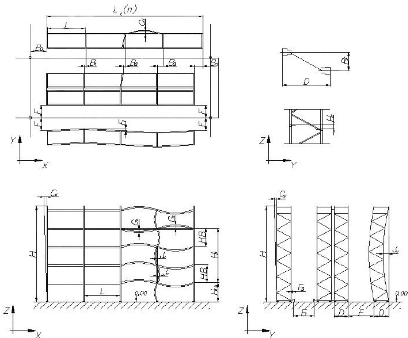
Рисунок 7 - Параметры, подлежащие контролю в ненагруженном состоянии системы
