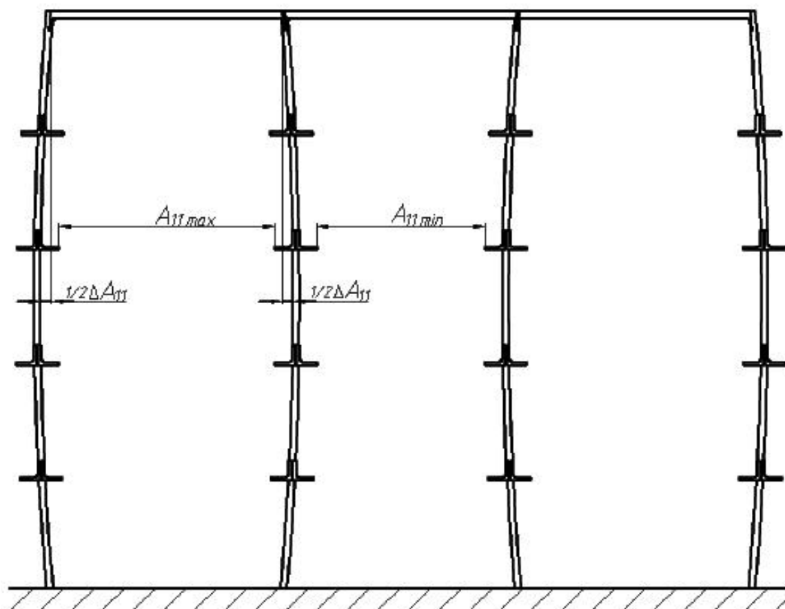
Рисунок 10 - Отклонение стоек от вертикальной плоскости внутри канала
