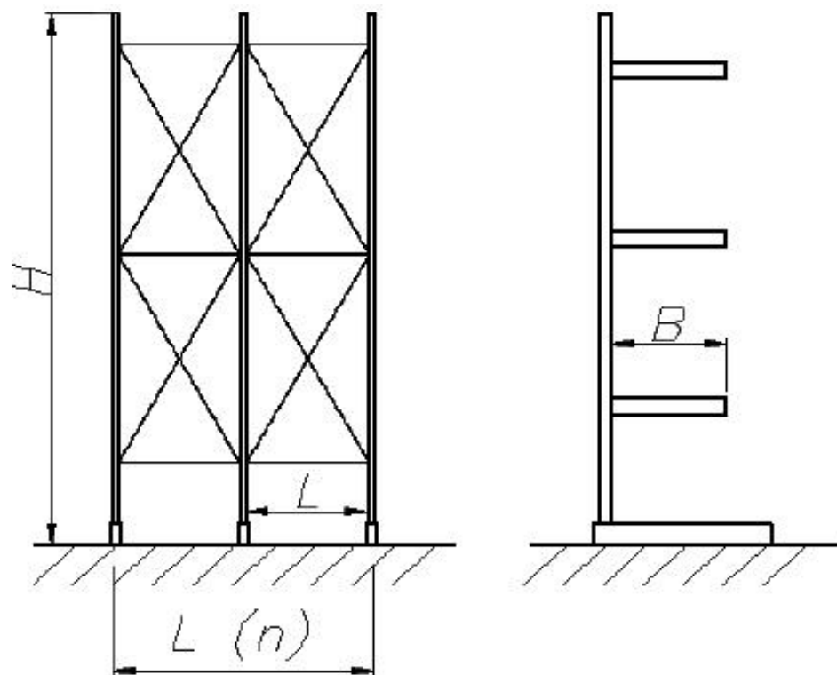
Рисунок 3 - Общий вид консольного стеллажа
