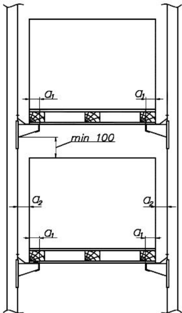
Рисунок 8 - Размещение груза относительно опорных профилей (грузонесущих направляющих)
