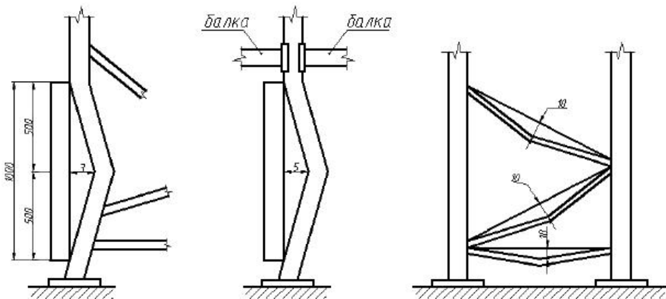
Рисунок Б.1 - Максимально допустимые значения деформации элементов
